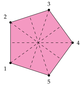
fr^2 = r^3 f
