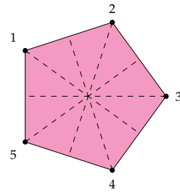
fr^3 = r^2 f
